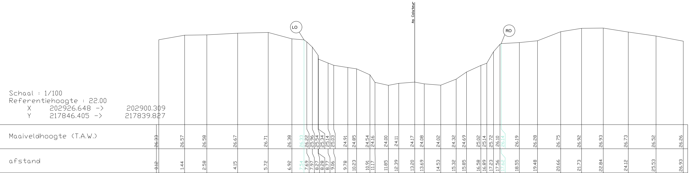
Pad ref: A.8.24.1 Dwarsprofiel 15
