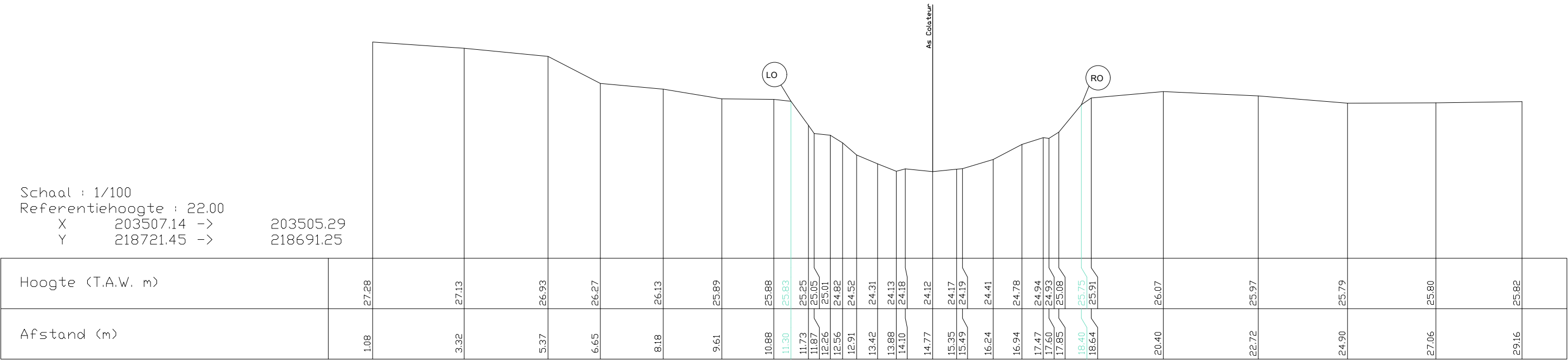
Pad ref: A.8.24.1 Dwarsprofiel 18
