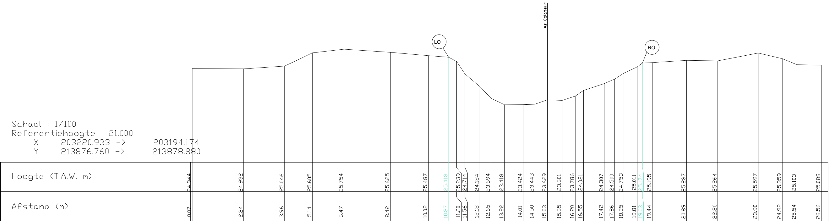
Pad ref: A.8.24.1 Dwarsprofiel 2
