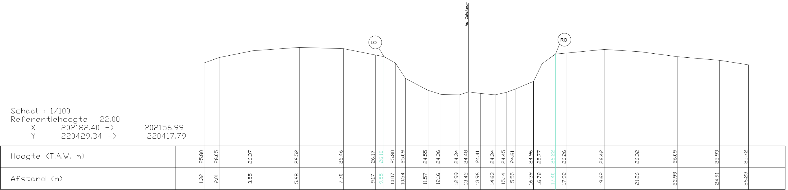
Pad ref: A.8.24.1 Dwarsprofiel 24
