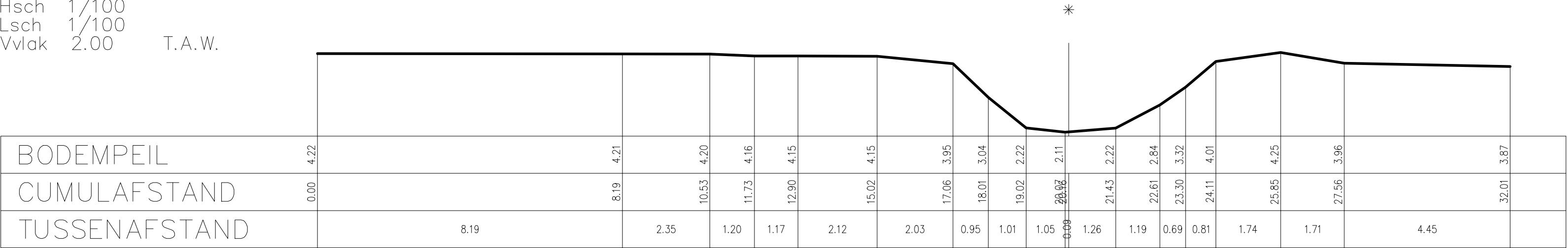
DWARSPROFIEL 147
