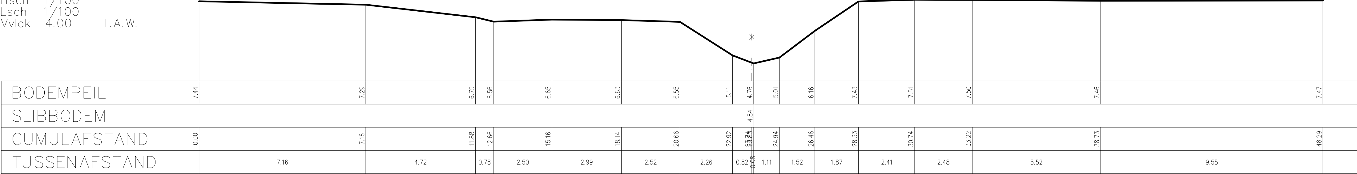
DWARSPROFIEL 244
