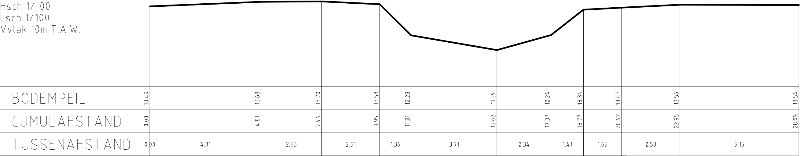
DWARSPROFIEL 176
