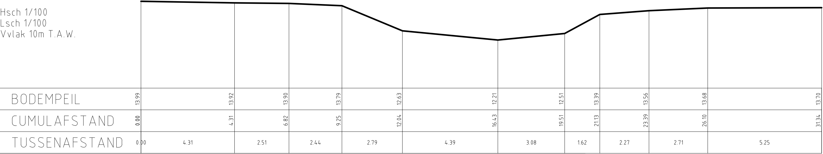
DWARSPROFIEL 177
