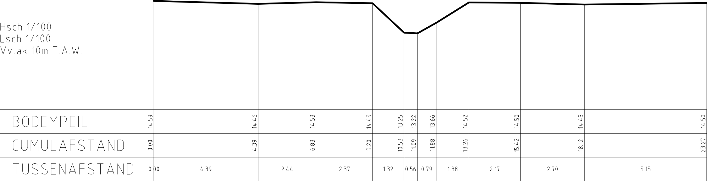
DWARSPROFIEL 180
