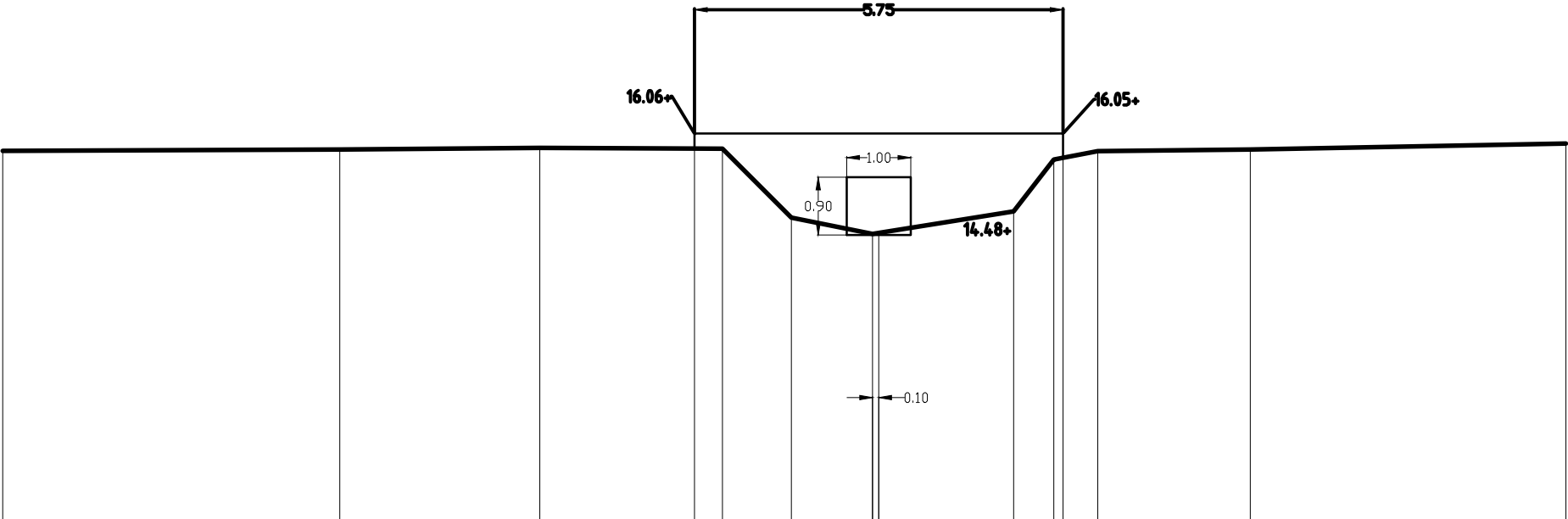
DWARSPROFIEL 188
