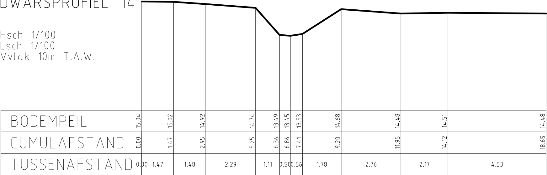
DWARSPROFIEL 14
