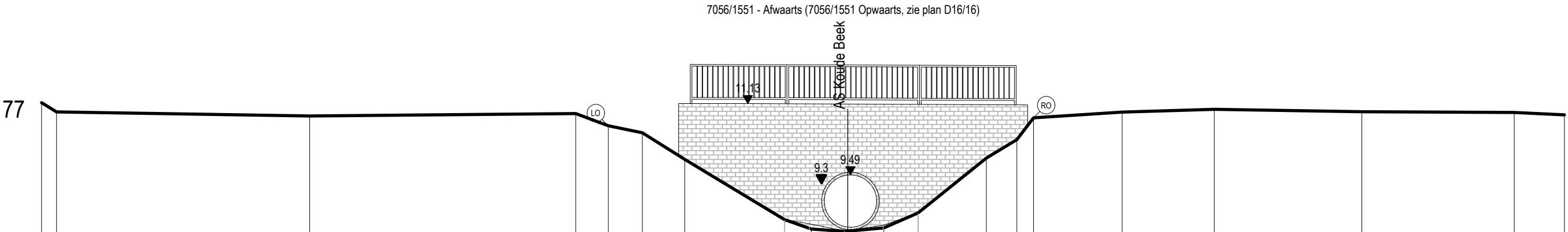
DWARSPROFIEL 77
