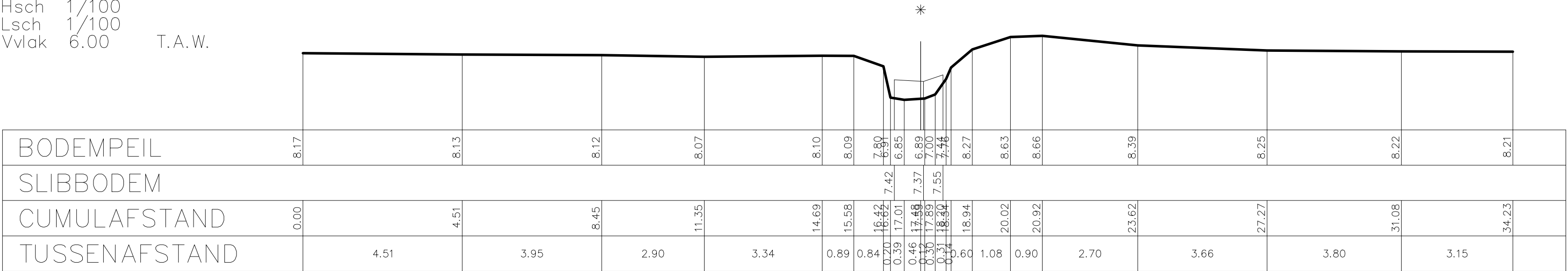
DWARSPROFIEL 12
