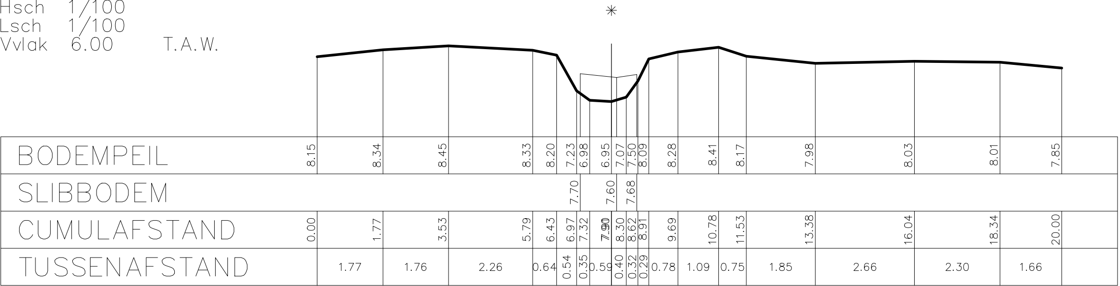
DWARSPROFIEL 20
