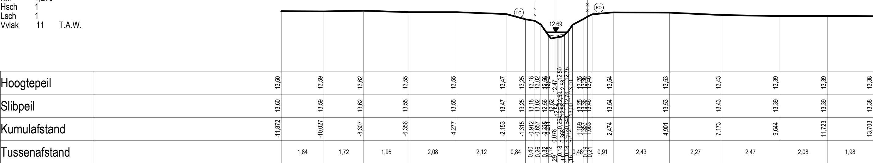
DWARSPROFIEL 31
