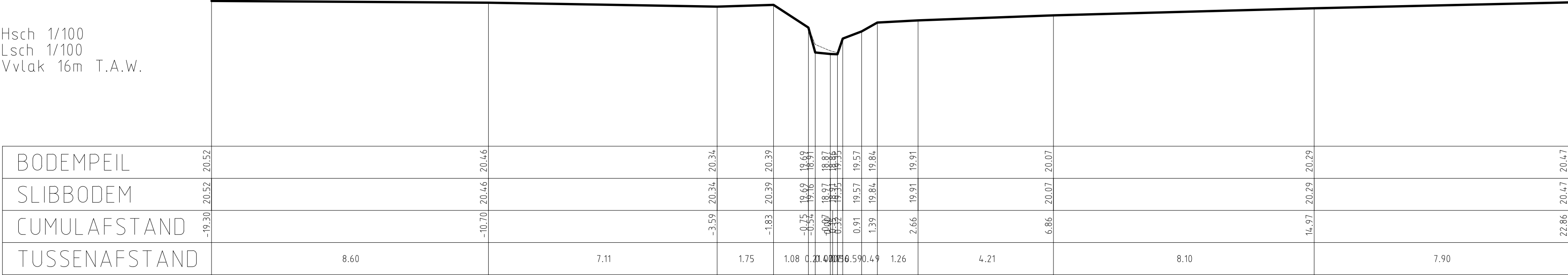
DWARSPROFIEL 104
