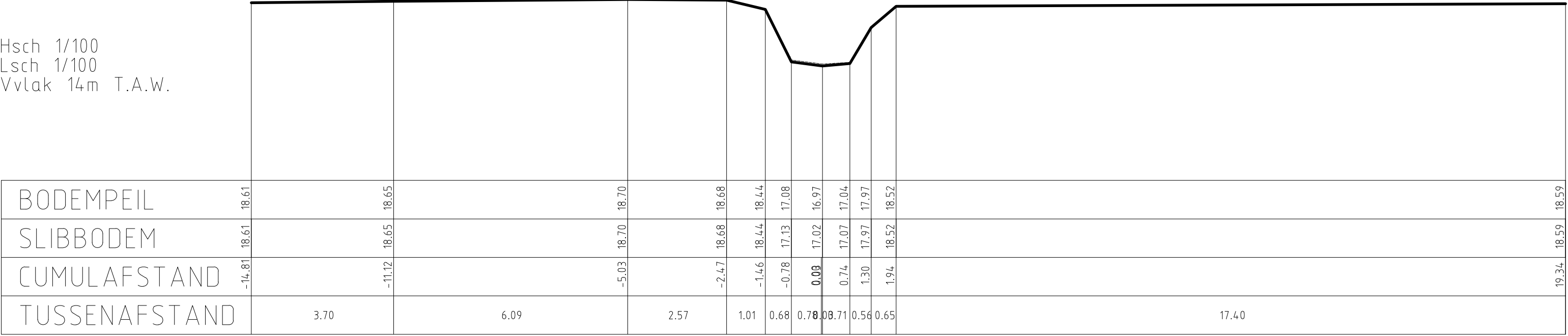
DWARSPROFIEL 96
