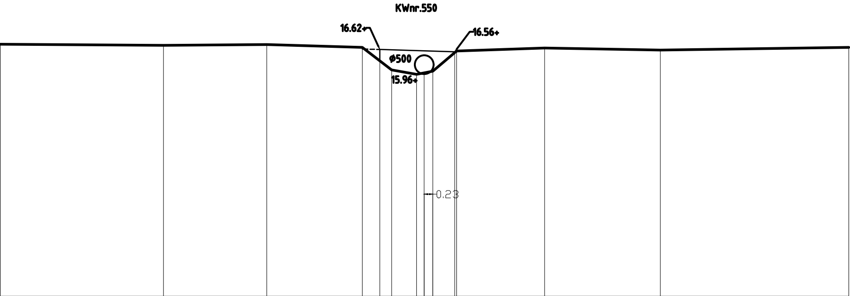
DWARSPROFIEL 203
