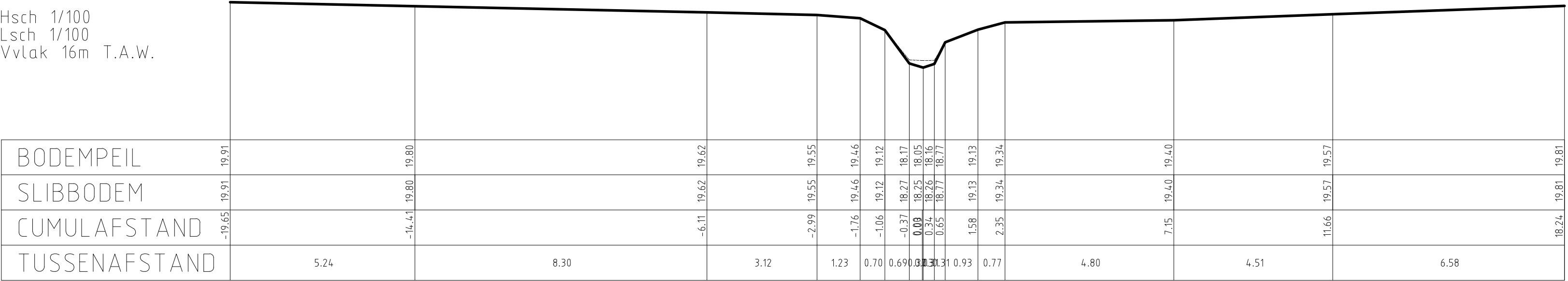
DWARSPROFIEL 18
