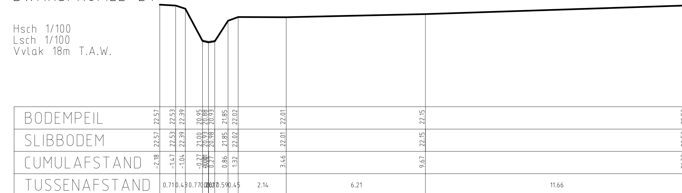
DWARSPROFIEL 24
