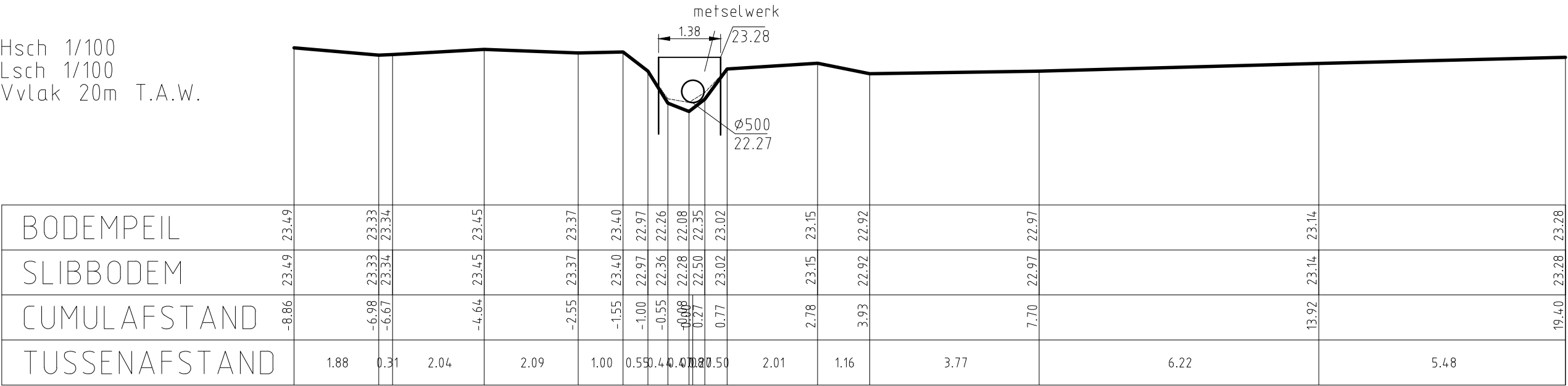
DWARSPROFIEL 28 K2: VA
