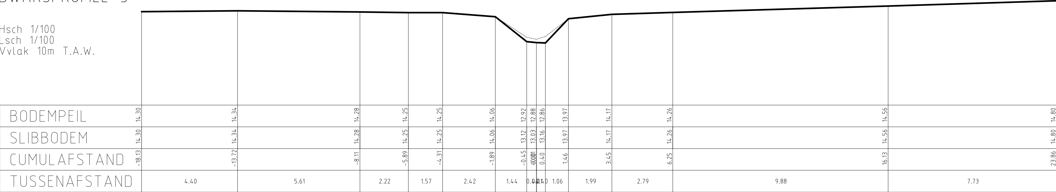
DWARSPROFIEL 5
