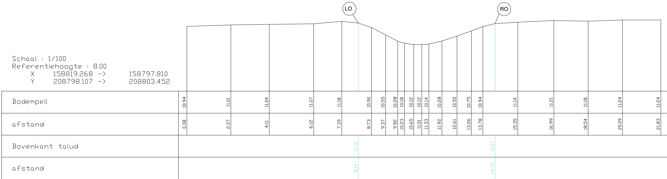
Pad ref: A.3.13.1_Dwarsprofiel 38
