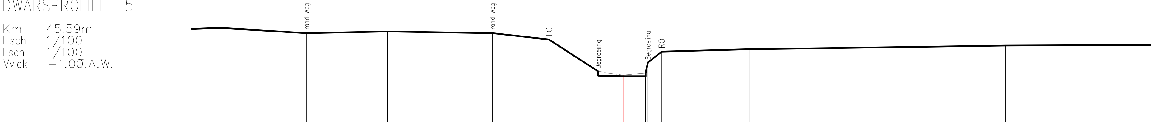
DWARSPROFIEL 5
