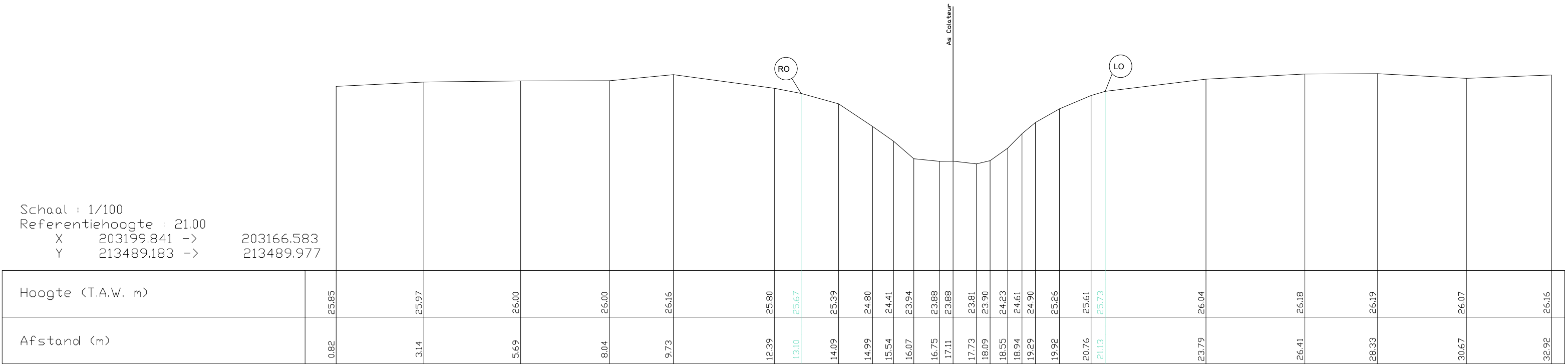
Pad ref: A.8.24.1 Dwarsprofiel 2
