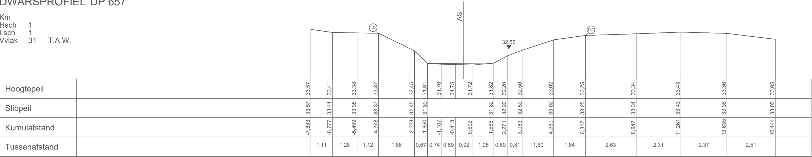
DWARSPROFIEL DP 657
