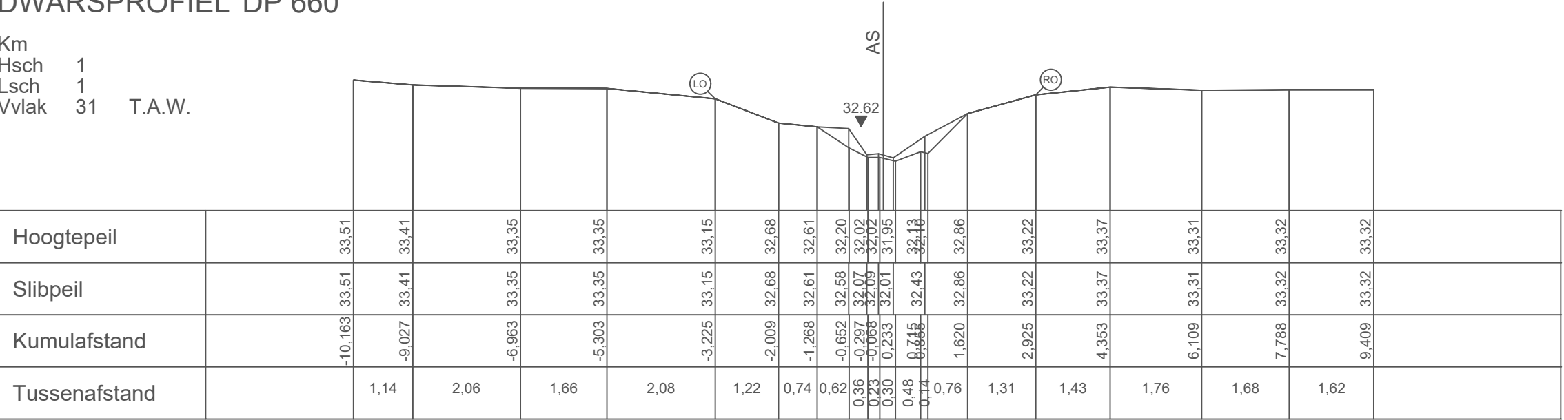
DWARSPROFIEL DP 660
