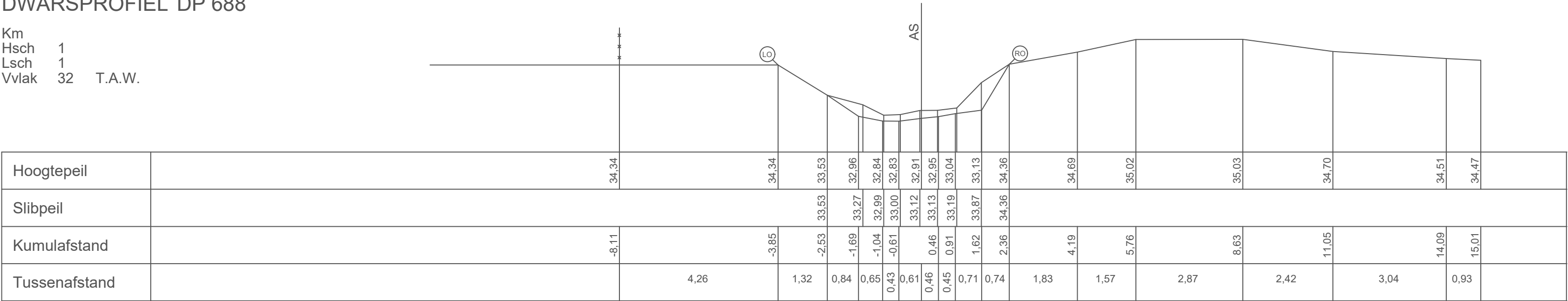
DWARSPROFIEL DP 688
