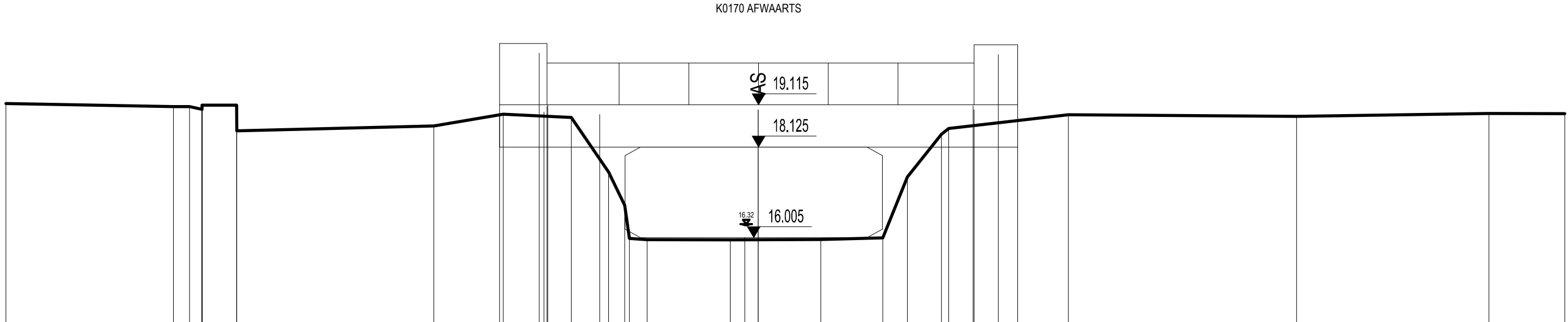
DWARSPROFIEL 23
