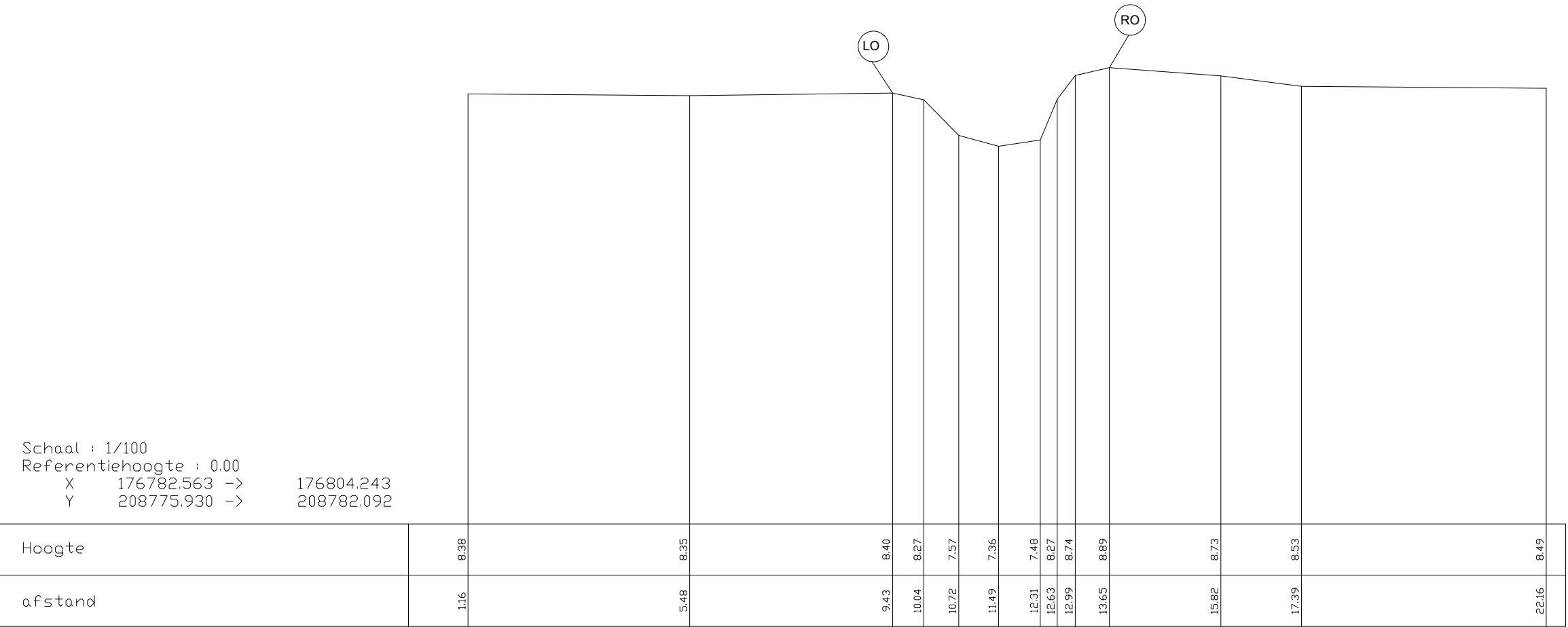
Pad ref: Dwarsprofiel 4
