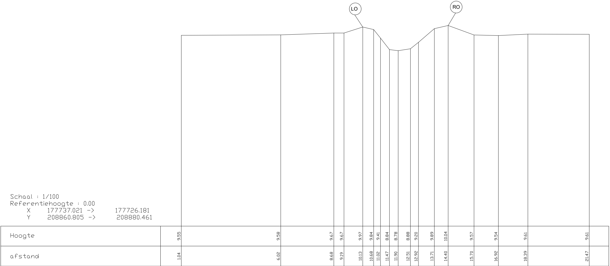
Pad ref: Dwarsprofiel 9
