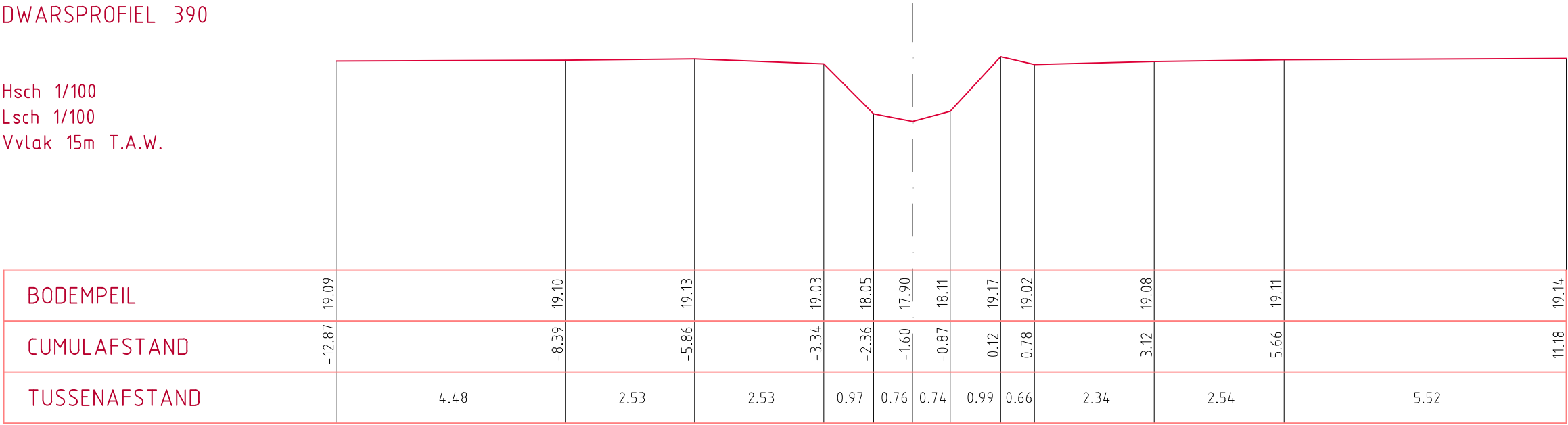
DWARSPROFIEL 390
