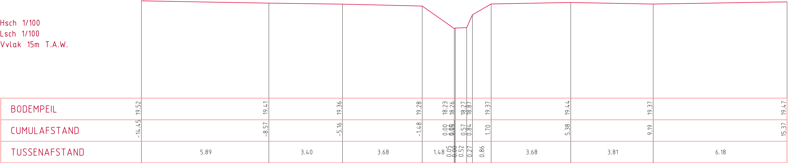
DWARSPROFIEL 393
