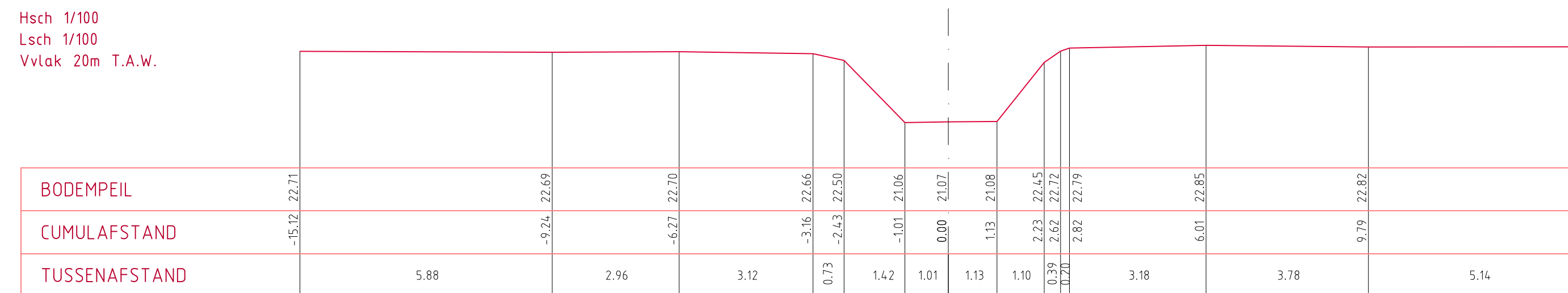
DWARSPROFIEL 413
