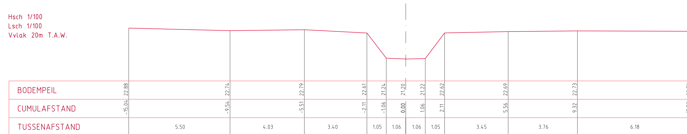
DWARSPROFIEL 414
