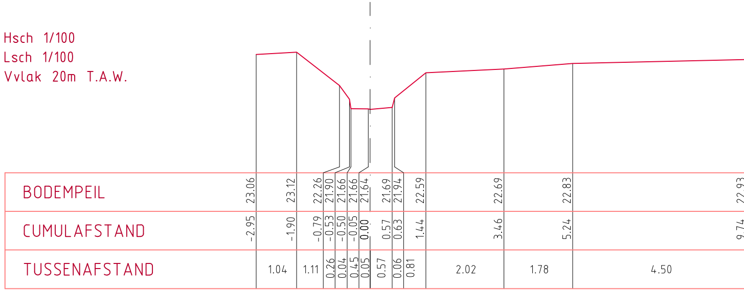
DWARSPROFIEL 418
