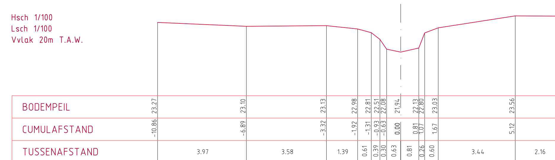
DWARSPROFIEL 420
