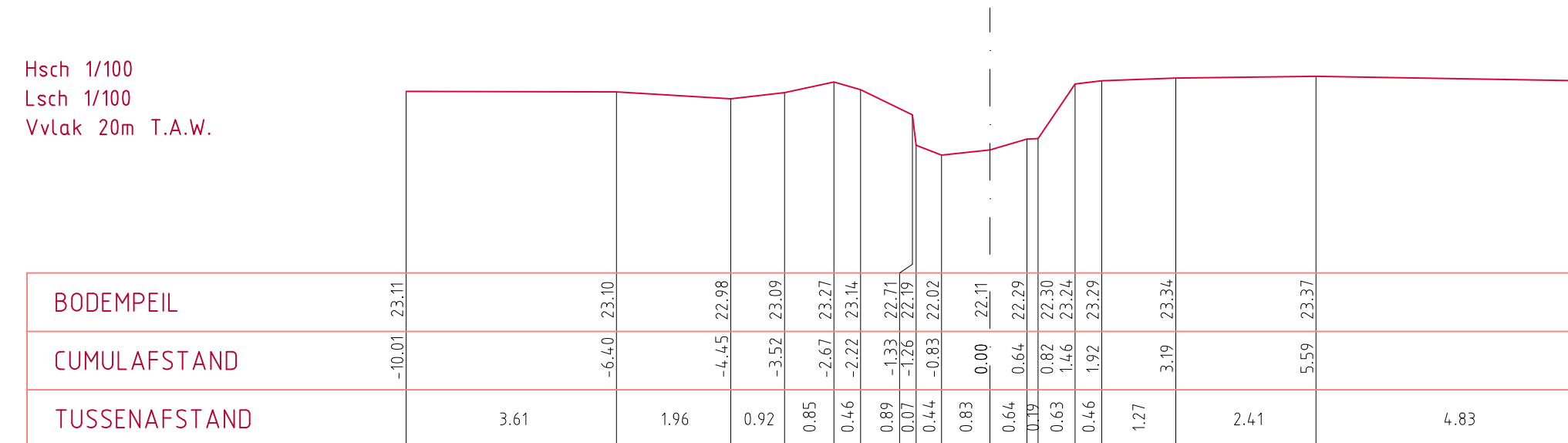
DWARSPROFIEL 421
