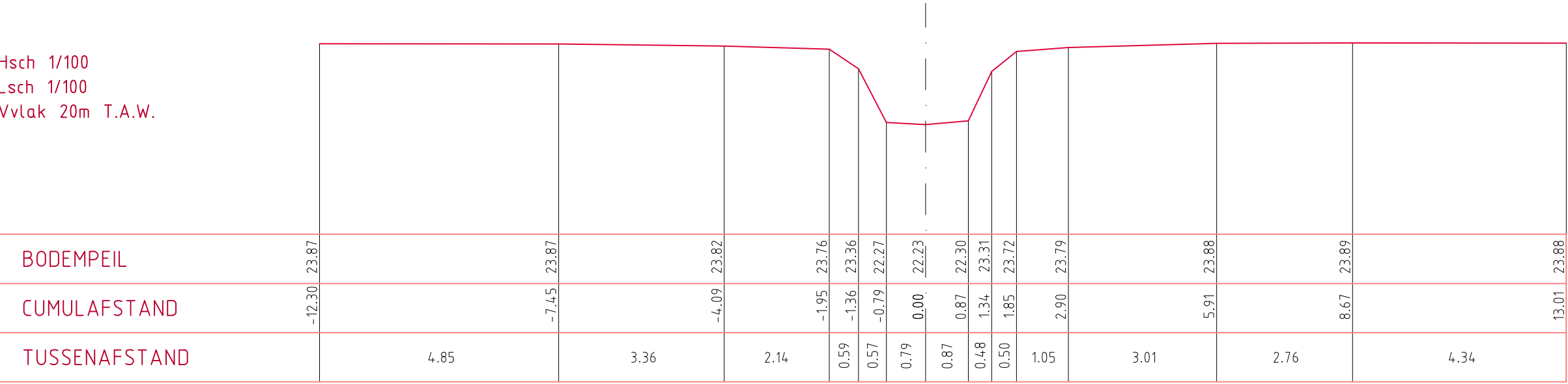
DWARSPROFIEL 422
