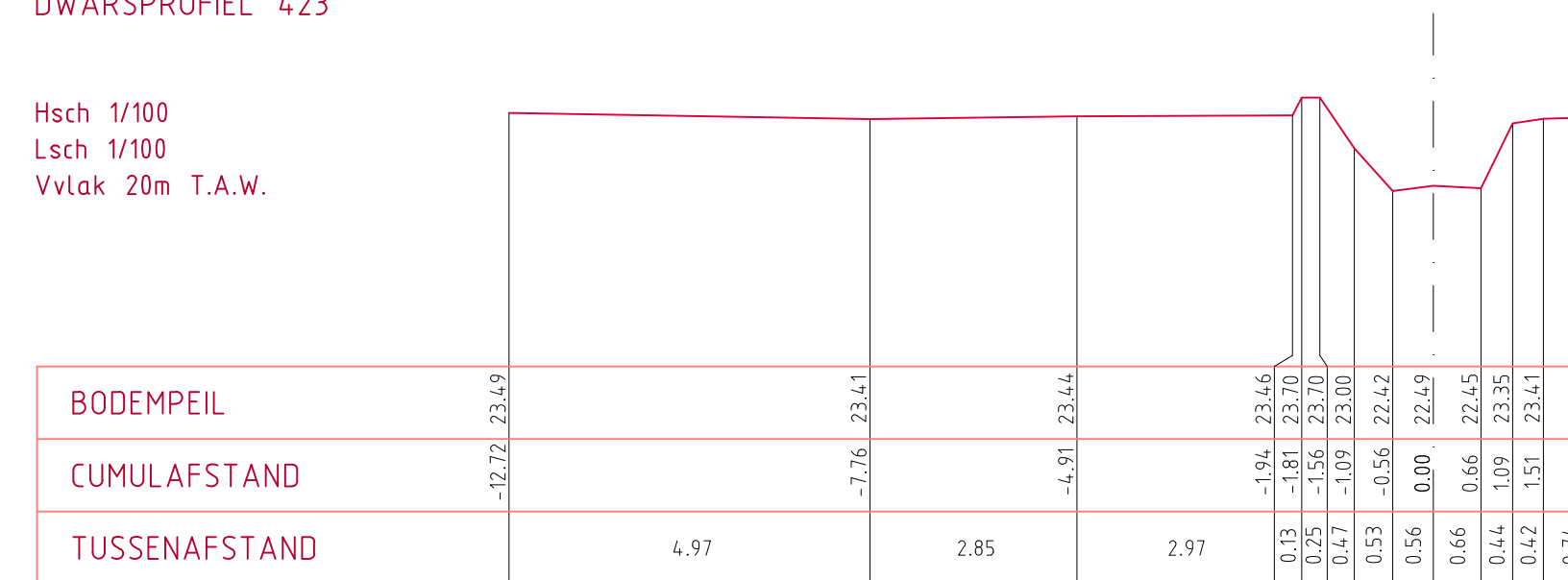
DWARSPROFIEL 423
