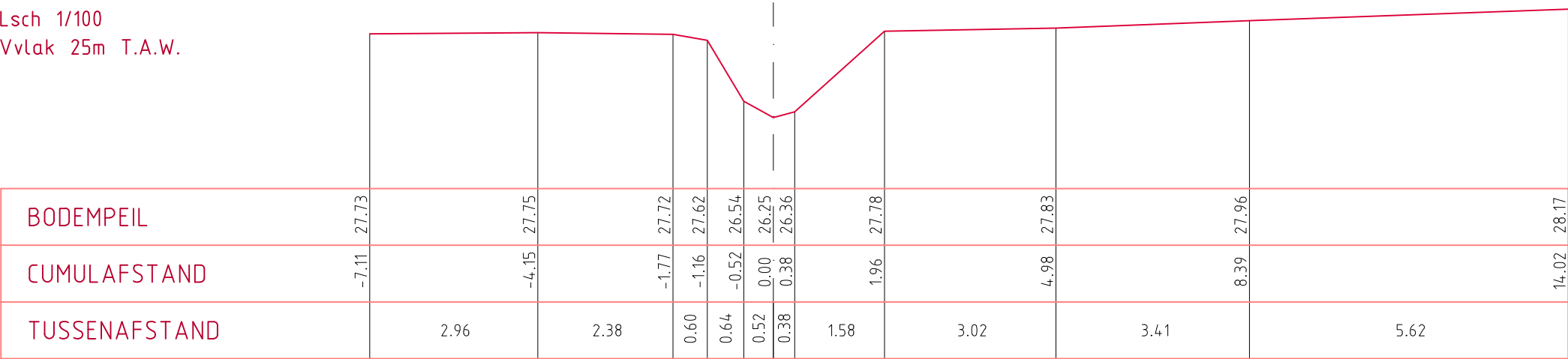
DWARSPROFIEL 449
