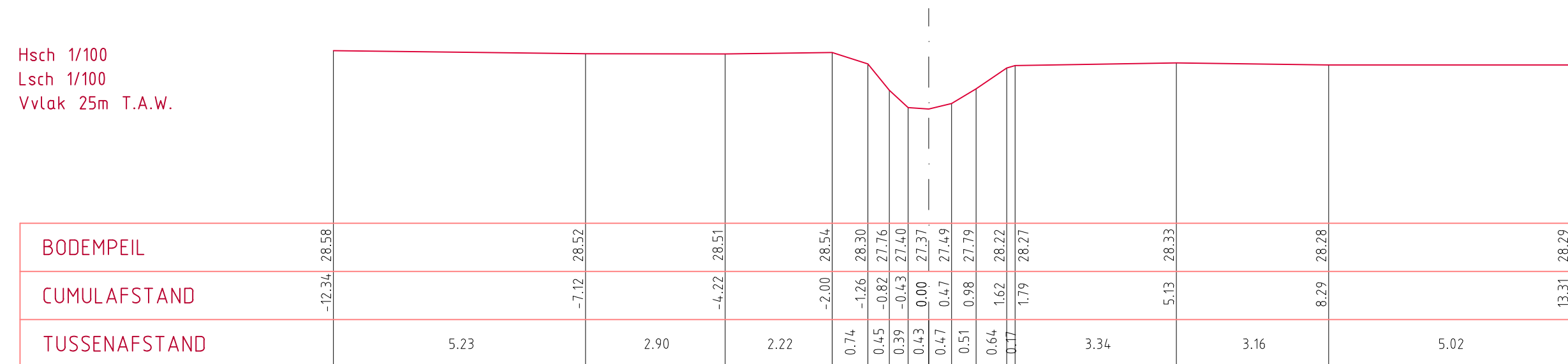
DWARSPROFIEL 451
