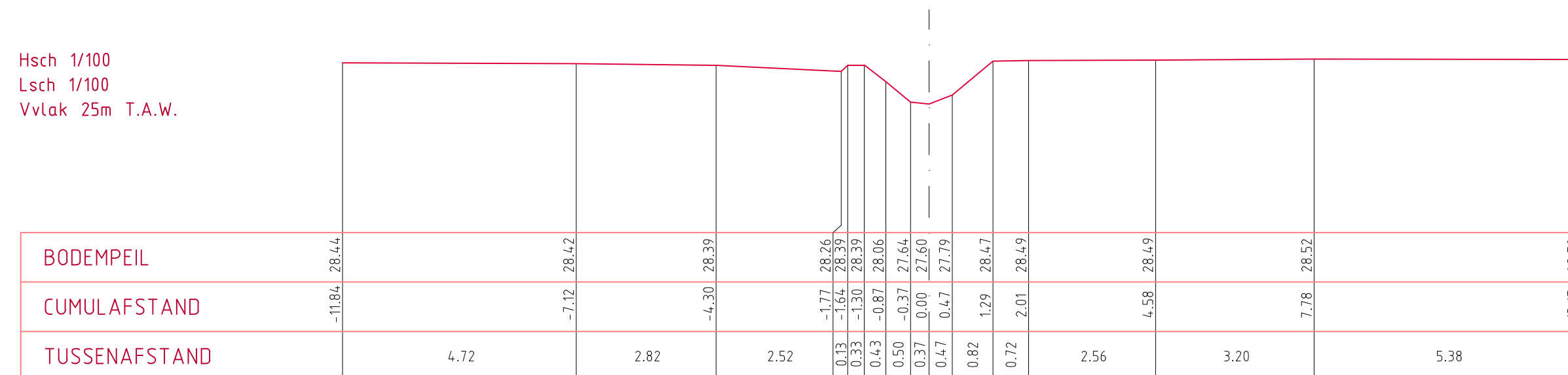
DWARSPROFIEL 453
