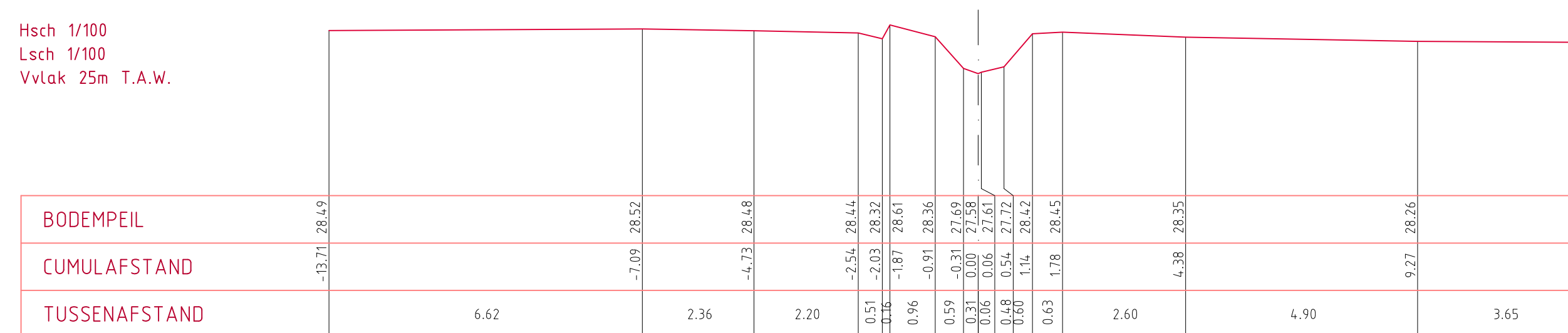
DWARSPROFIEL 454
