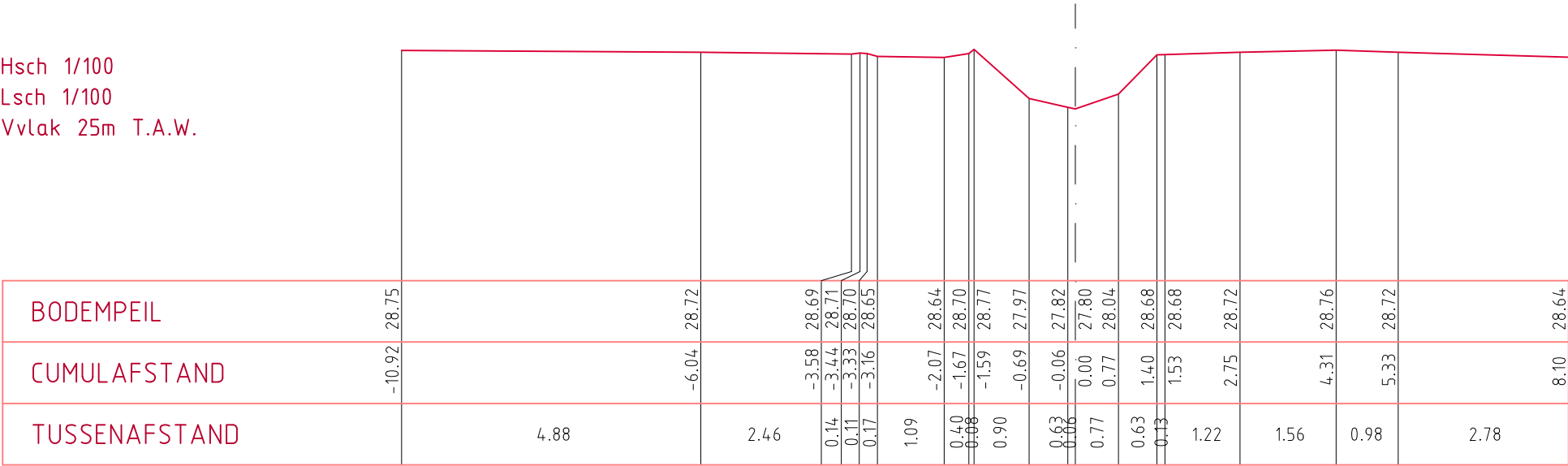
DWARSPROFIEL 456
