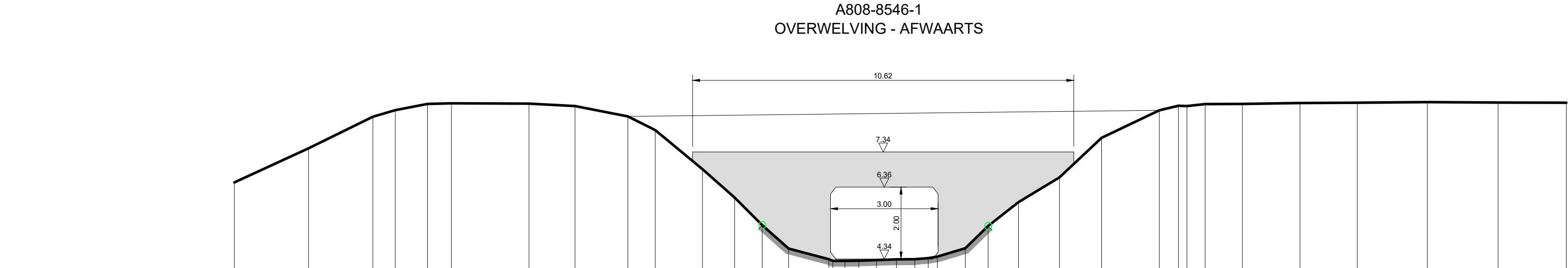
DWARSPROFIEL 1
