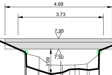
A808-8555-31 BRUG - OPWAARTS
