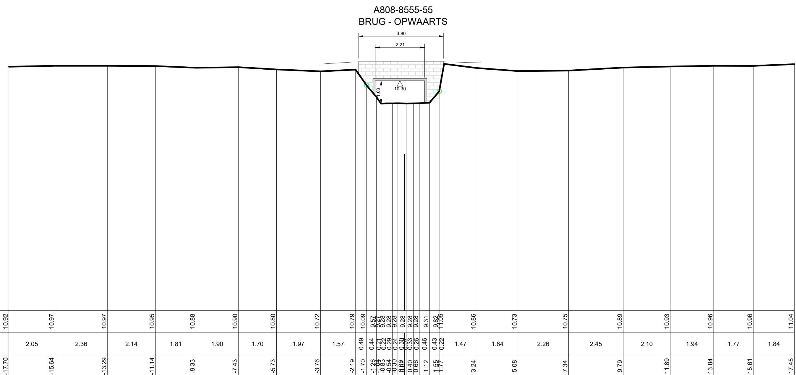
DWARSPROFIEL 290
