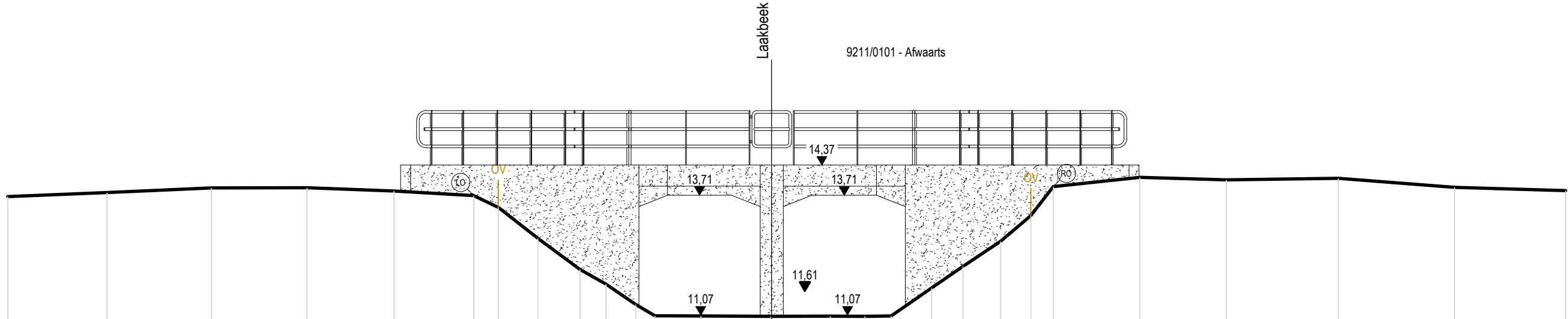
DWARSPROFIEL 19
