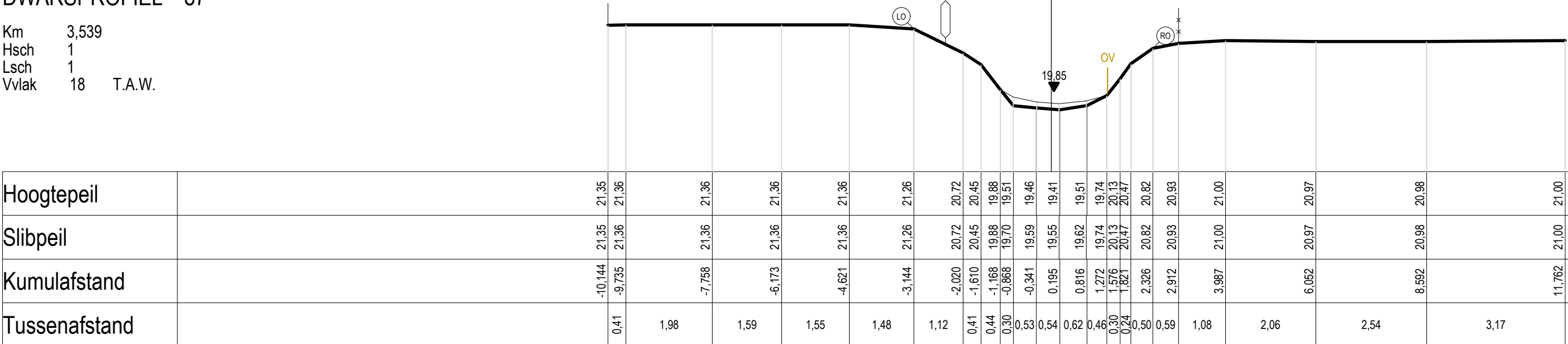
DWARSPROFIEL 87
